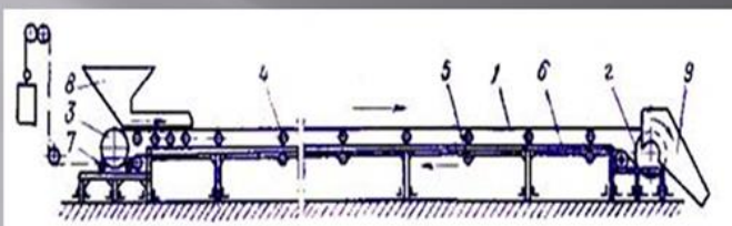
Схема стрічкового конвеєра: 1 – стрічка; 2 – приводний барабан; 3 – натяжний барабан; 4 – роликові опори; 5 – роликові опори порожньої гілки; 6 – опірня рама; 7 – натяжний пристрій; 8 – завантажувальна лійка; 9 – розвантажувальний жолоб
